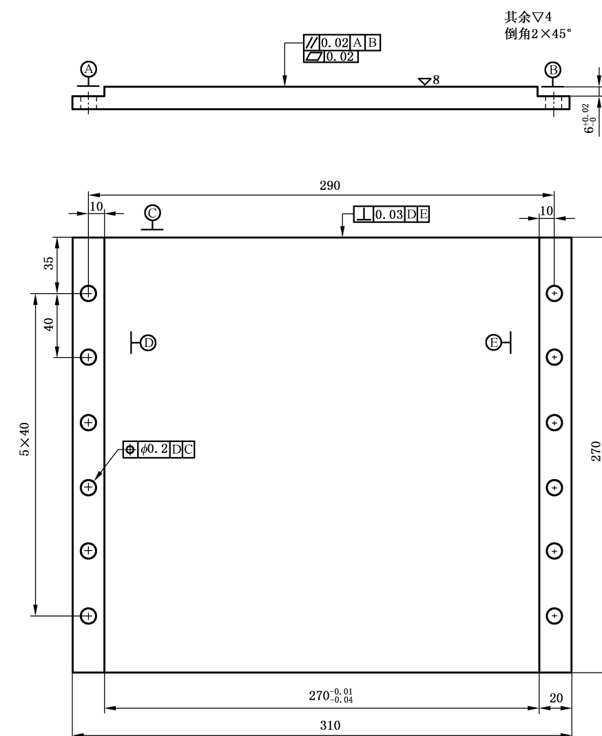
图 3b 压板尺寸及要求
